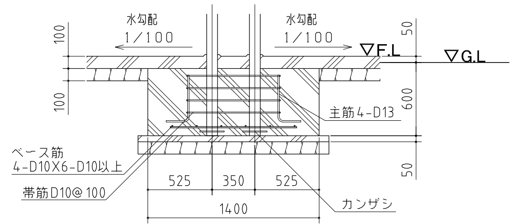
A-A' 断面
